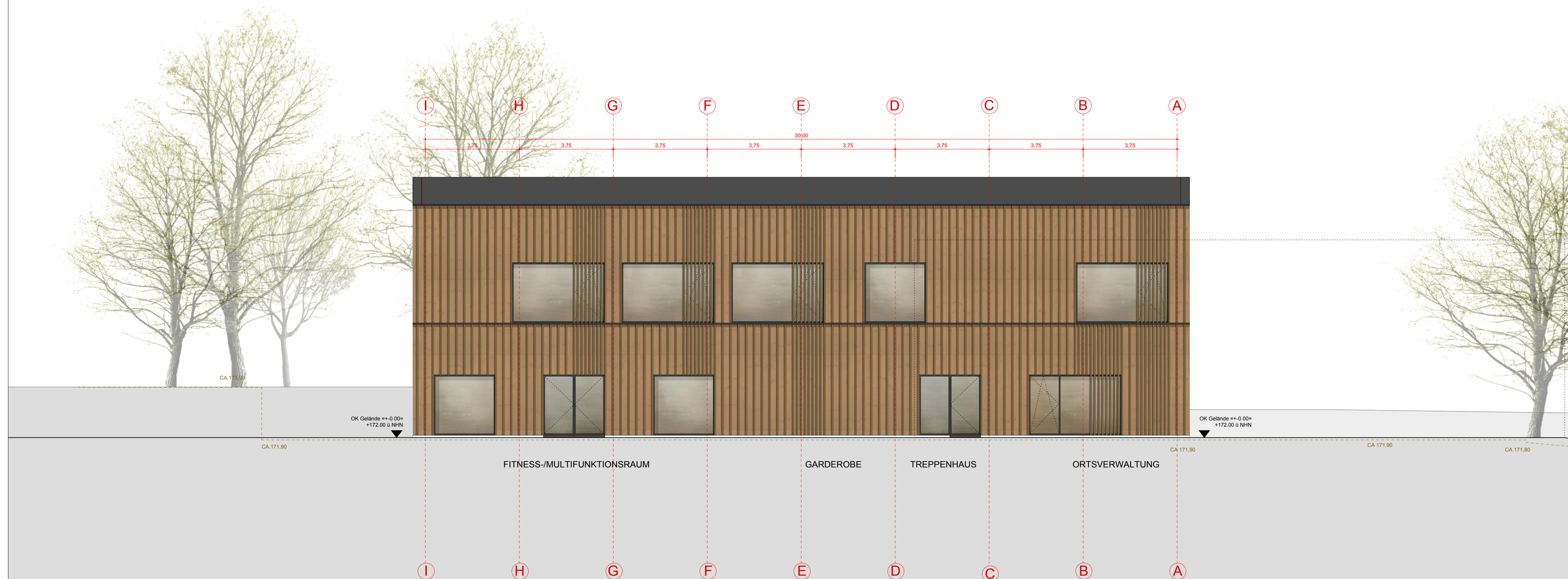
ANSICHT NORD-NORDOST
