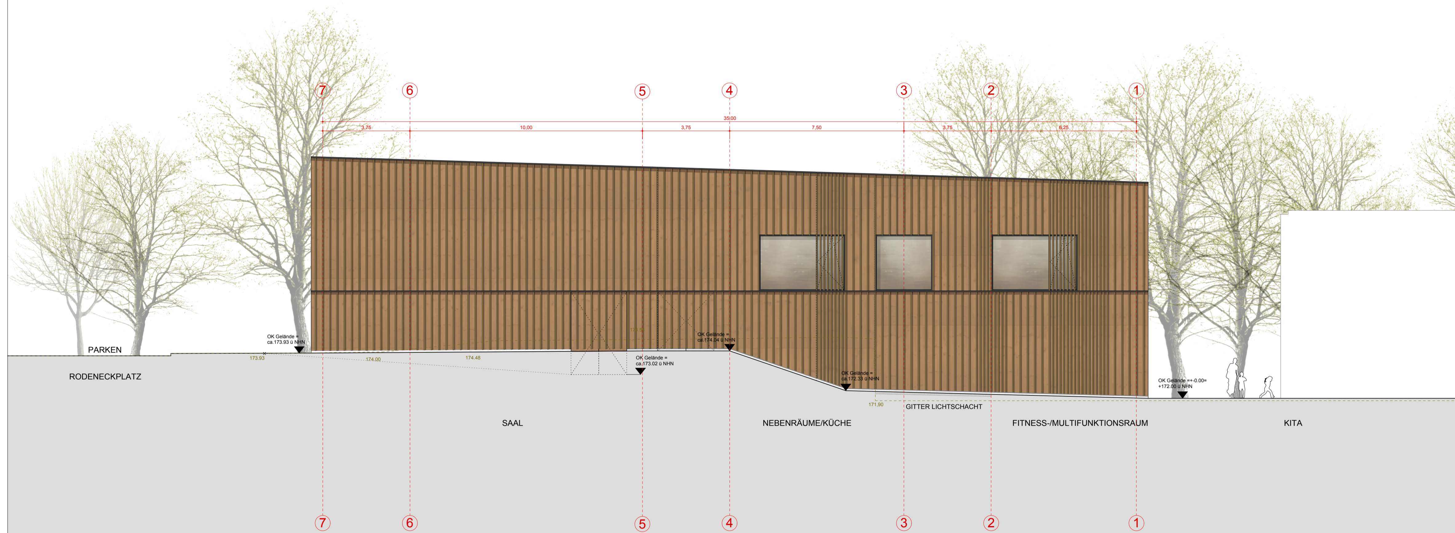
ANSICHT OST-SÜDOST
